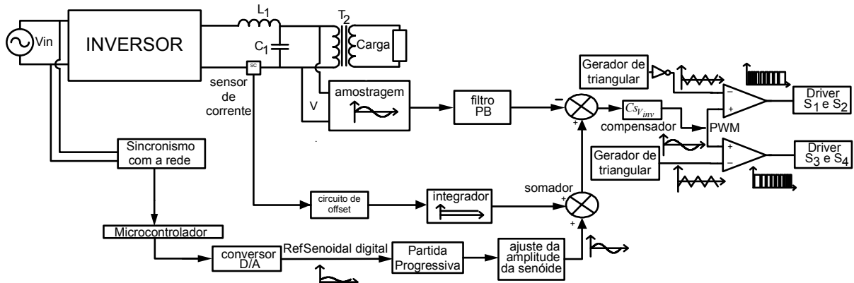
Figura 2.39 – Circuito de controle completo do inversor
