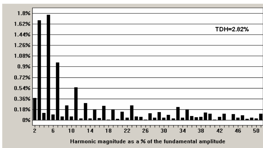
Figura 5.31 - Análise harmônica da tensão de saída da UPS.
