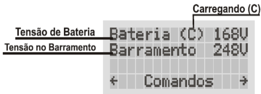
Figura 4.20 – Tela com UPS em modo bateria.
