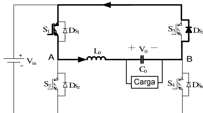
Figura 2.6 - Segunda etapa do semiciclo positivo.
