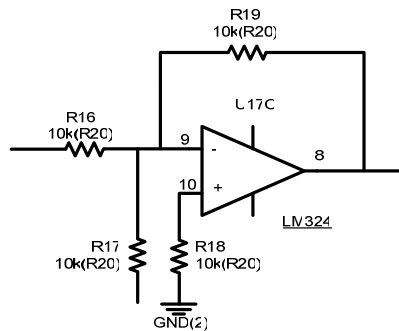
Figura 2.27 - Circuito somador.
