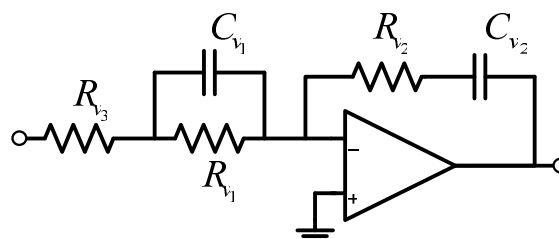
Figura 2.34 – Compensador PID.
