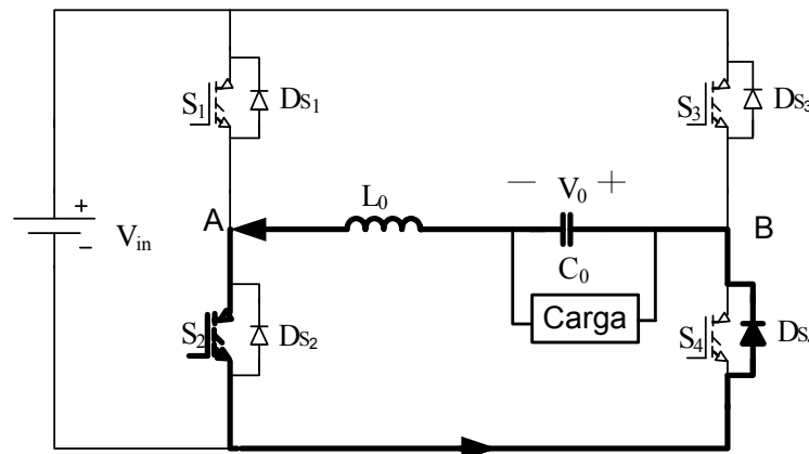
Figura 2.10 - Segunda etapa do semiciclo negativo.
