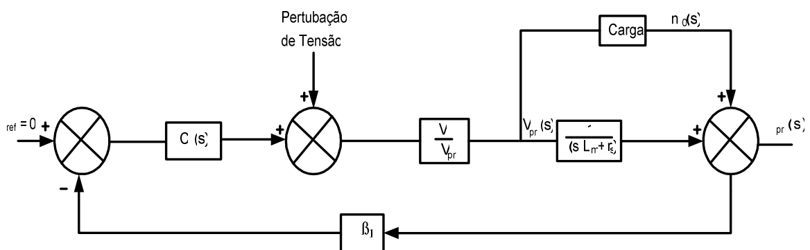
Figura 2.38 – Diagrama de blocos do da malha de corrente
